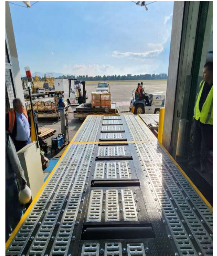
Sistema de rodillos por gravedad para movilización de pallets y contenedores aéreos
