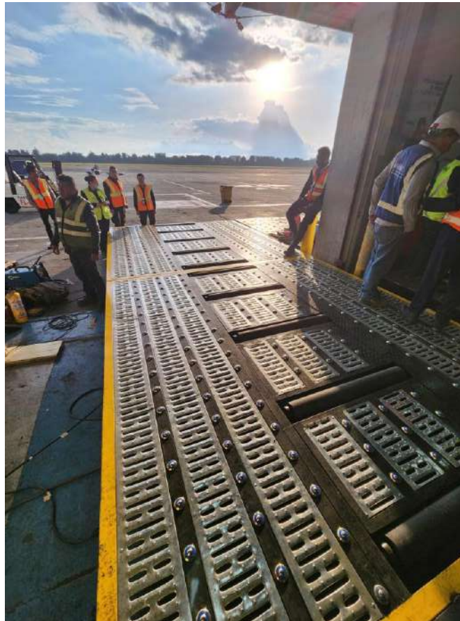
Sistema motorizado para movilización de pallets y contenedores aéreos
